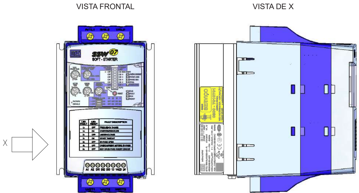
Figura 2.4 - Localização das etiquetas da Soft-Starter SSW-07
