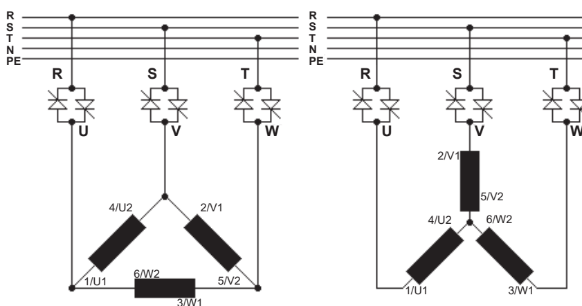
Figura 3.7 - Arrancador Suave SSW-07 con conexión padrón
