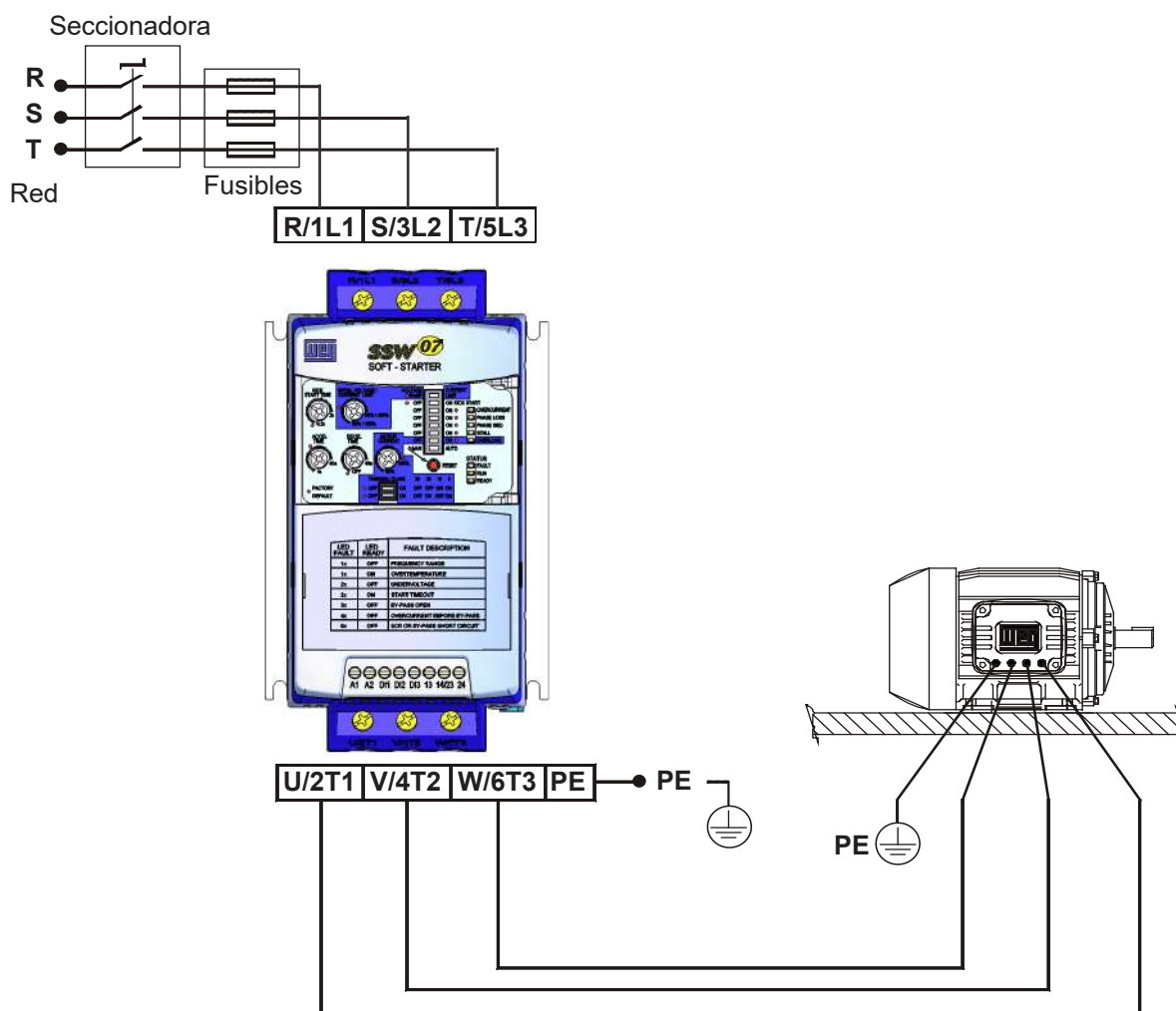
Figura 3.4 - Conexiones de potencia y de puesta a tierra para conexión estándar
