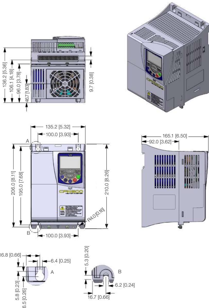
Figure B.7: Inverter dimensions in mm [in] - frame size C Figura B.7: Dimensiones del convertidor en mm [in] - tamaño C Figura B.7: Dimensões do inversor em mm [in] - mecânica C
