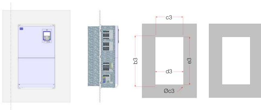
(c) Flange mounting - standard inverter (c) Montaje en flange - convertidor estándar (c) Montagem em flange - inversor padrão
