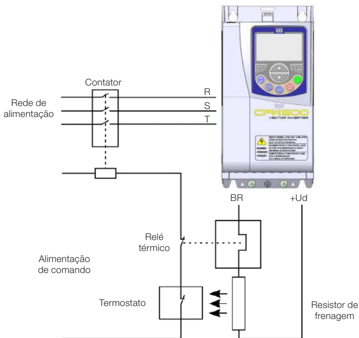
Figura 3.2: Conexão do resistor de frenagem
