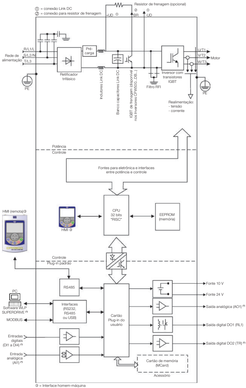
Figura 2.3: Blocodiagrama da CFW500 para mecânicas F e G
