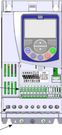
Frame Size D (200 V line) Tamaño D (línea 200 V) Mecânica D (linha 200 V)
