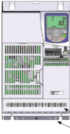
Frame Size D (200 V line) Tamaño D (línea 200 V) Mecânica D (linha 200 V)
