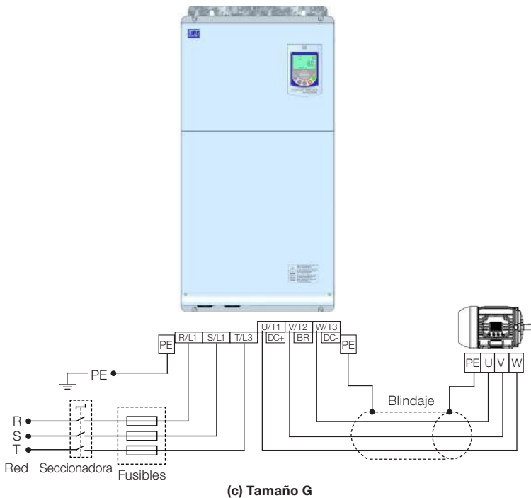
Figura 3.1: (a) a (c) Conexiones de potencia y aterramiento
