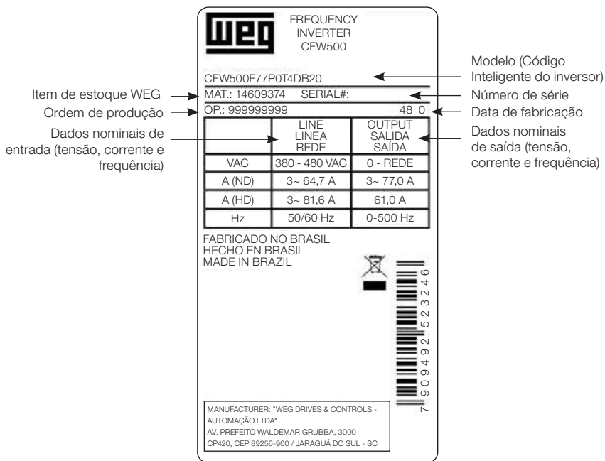
b) Etiqueta lateral do CFW500 para as mecânicas F e G
