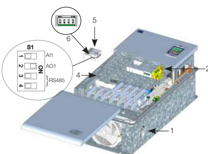
Frame Size G Tamaño G Mecânica G
